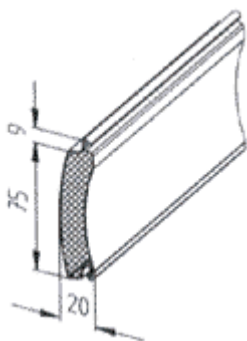
Profil 75 E, 75 D, 75 S
