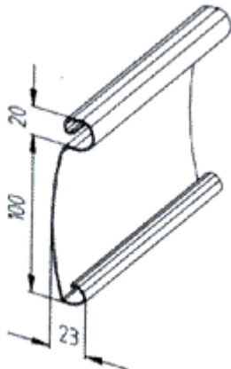
Profil 100 einw.
